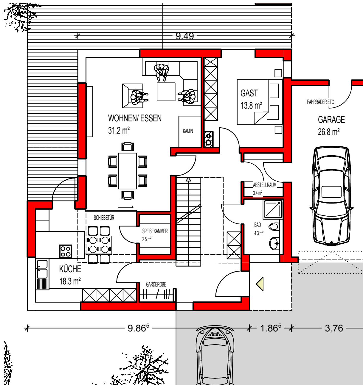
Grundriss Erdgeschoss
