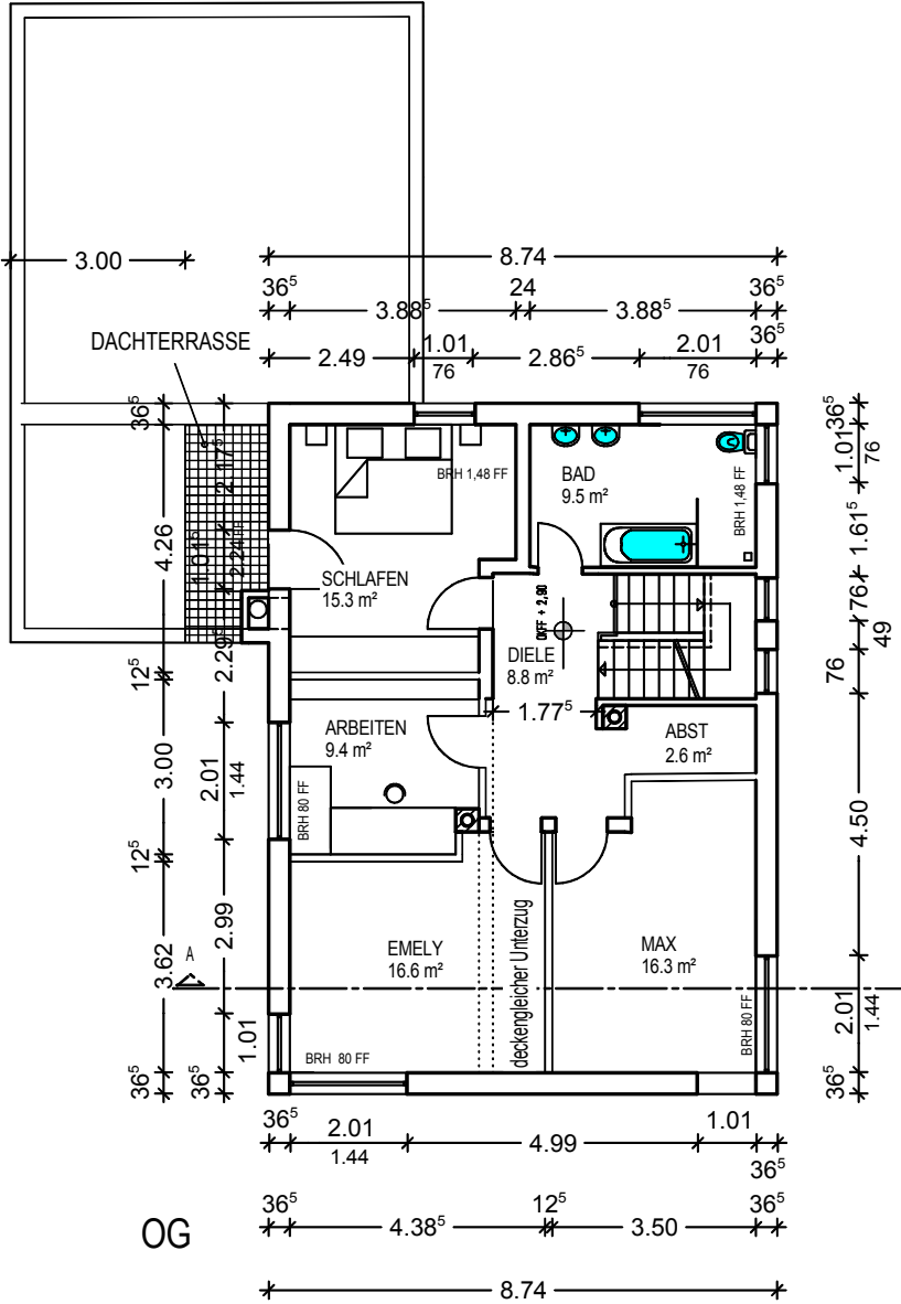
Grundriss Obergeschoss
