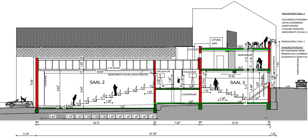
Schnitt A_A
