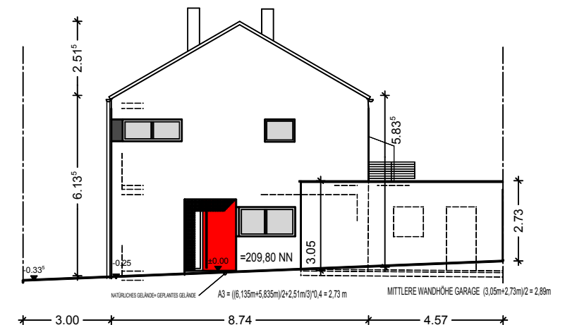
Strassenansicht
