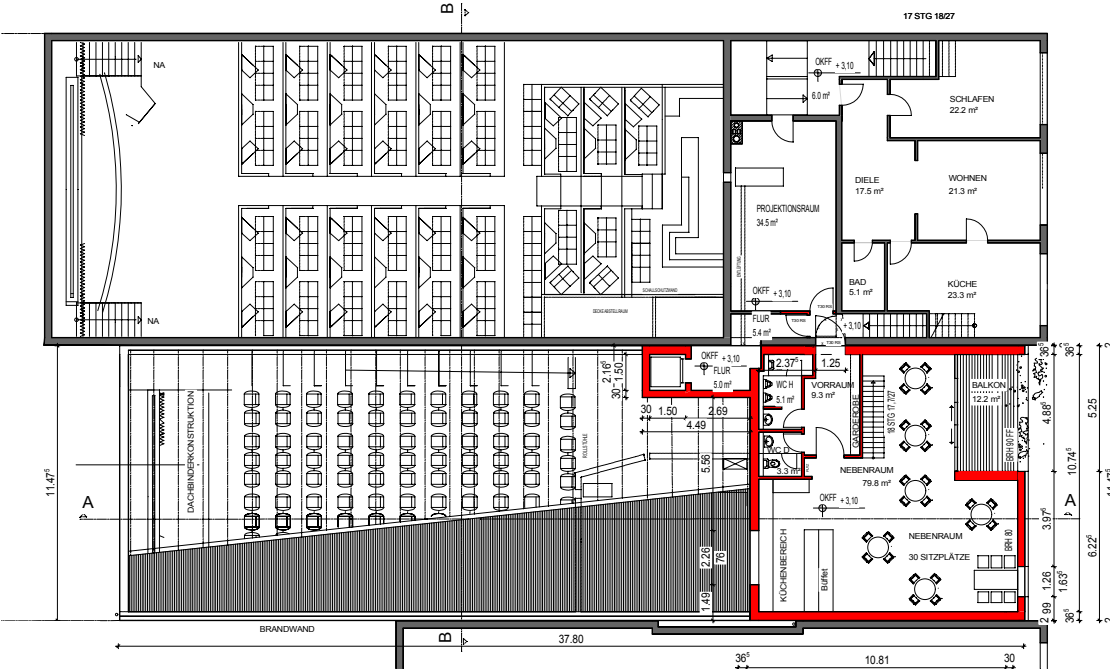
Grundriss Obergeschoss
