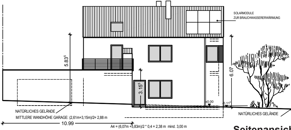
Seitenansicht rechts
